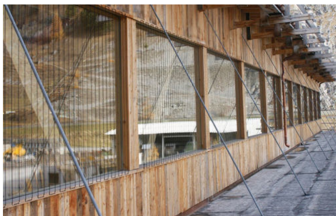
Nach wiederholtem Vogelanprall an den spiegelnden Fenstern einer Werkhalle in S-charnf wurden nachträglich im Abstand von 8–10 cm schwarze Nylo-schnüre gespannt. Im Anschluss an die Nachrüstung wurden keine Vogelkollisionen mehr dokumentiert.
